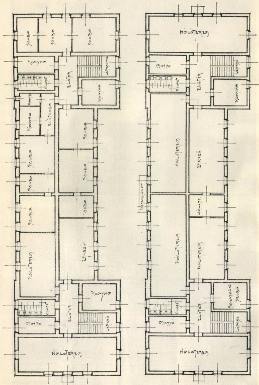
Koestlin L. és Társai piskólagár munkásothton-épületének földszinti és emeleti alaprajza (779. laphoz).
