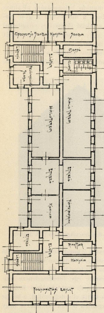
Koestlin L. és Társai piskótagyárában lévő munkás-otthon alagsorának alaprajza (779. laphoz).
