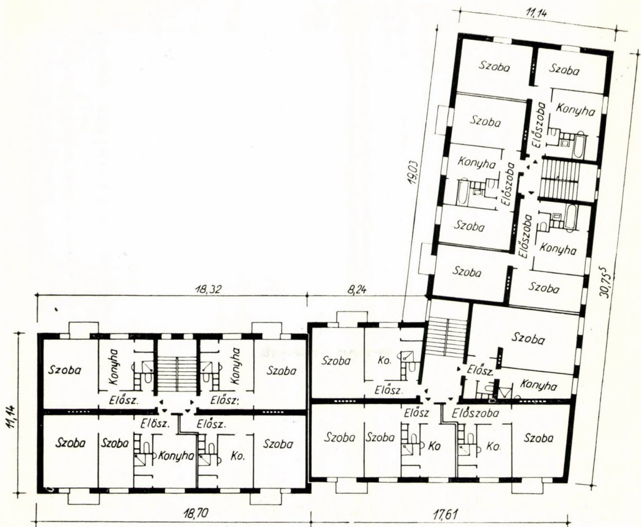
Győr, Kígyó utcai lakótelep, udvari homlokzat és alaprajz
